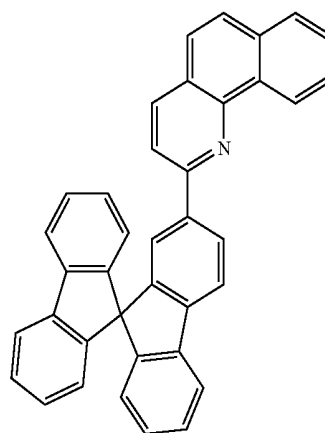
1174660-92-4 HBM-Ref
