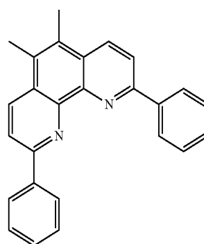
245068-13-7 TMM-Ref
