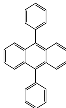
1499-10-1 SMB-Ref
